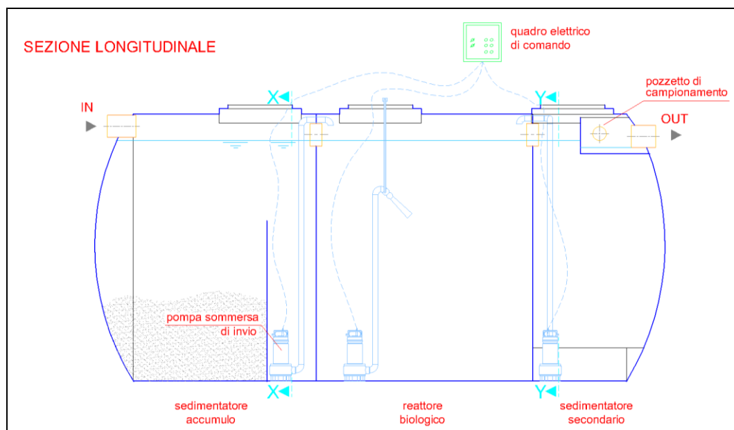
Figura 2 Mod. DFVA Sezione Longitudinale
