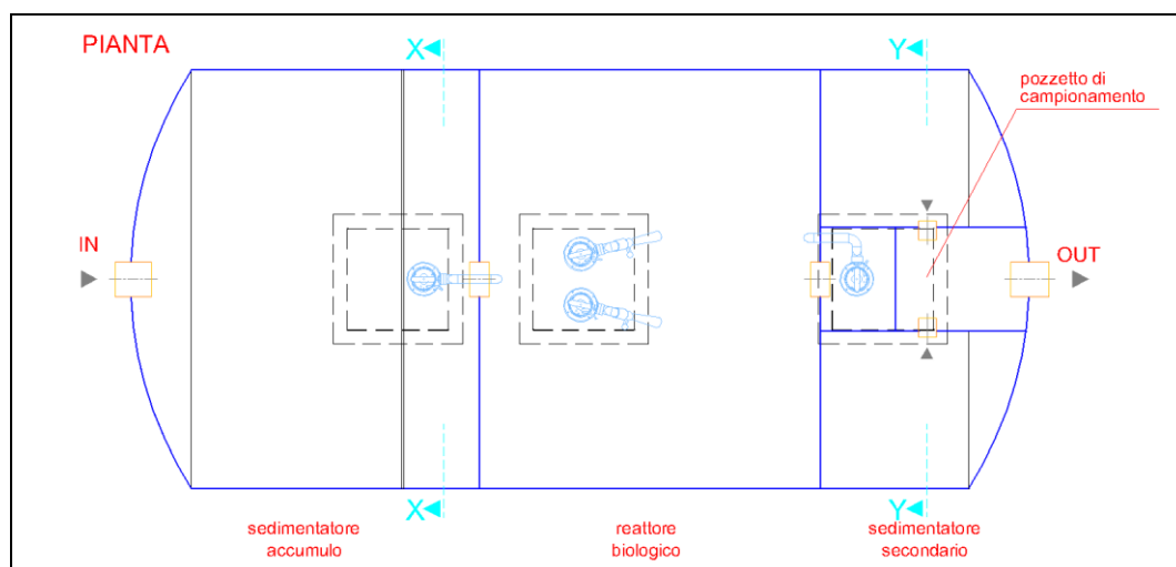
Figura 1 Mod. DFVA Pianta
