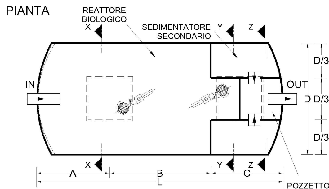
Figura 3 Mod. DFS Pianta
