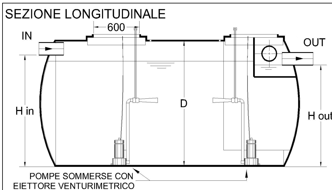
Figura 4 Mod. DFS Sezione Longitudinale
