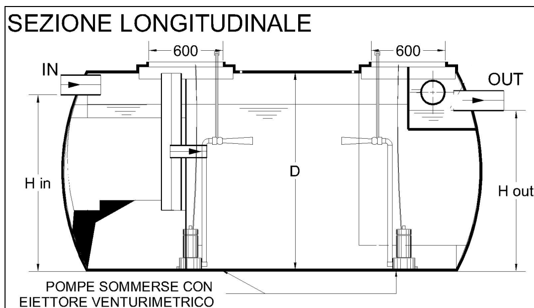
Figura 2 Mod. DF Sezione Longitudinale
