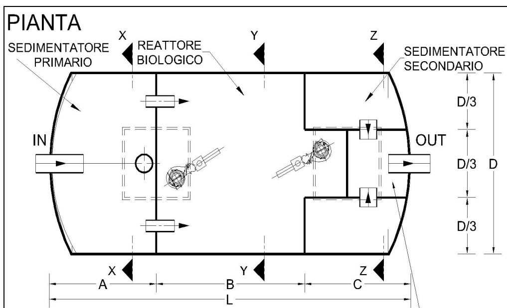
Figura 1 Mod. DF Pianta
