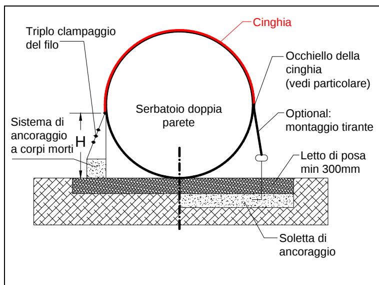
Figura 6 Disposizione delle cinghie di ancoraggio
