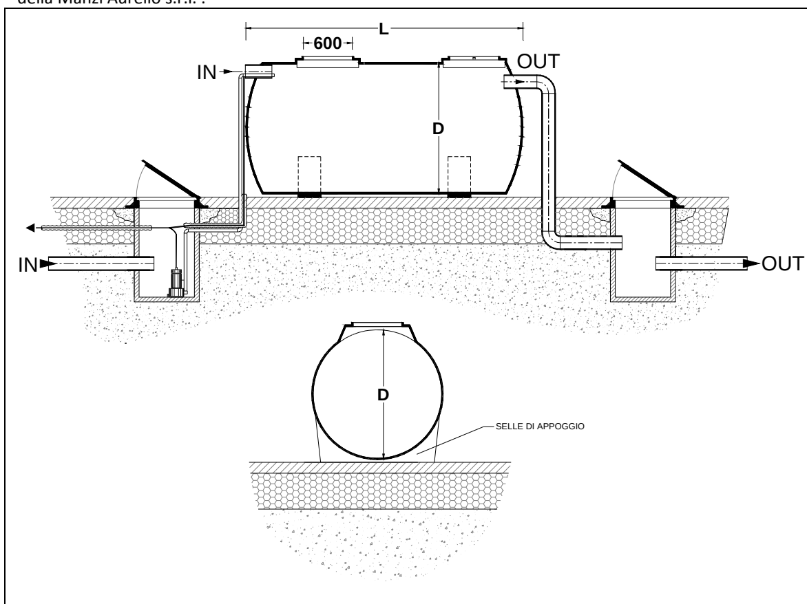
Figura 15 Installazione Fuori Terra
