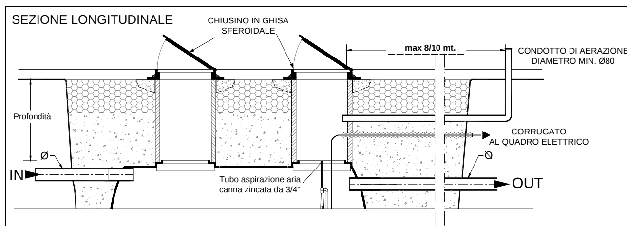
Figura 16 Realizzazione condotti aerazione
