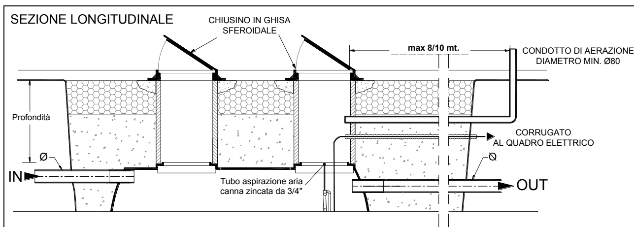
Figura 19 Realizzazione condotti aerazione con pompa sommersa
