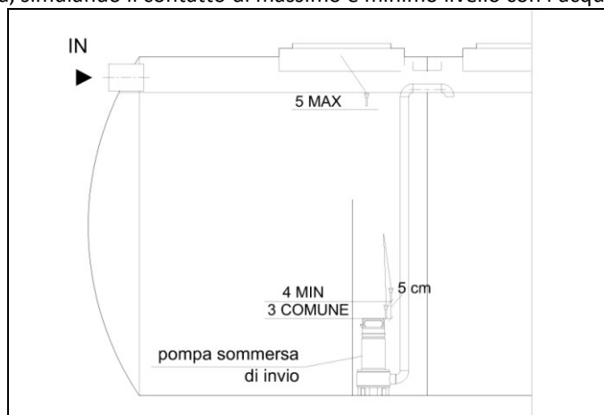
Figura 16 posizionamento sonde in settore accumulo per impianti mod. DFVA/DFVAF
