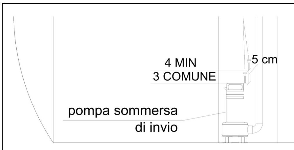
Figura 18 posizionamento sonde com e min
