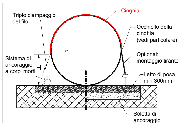
Figura 6 Disposizione delle cinghie di ancoraggio
