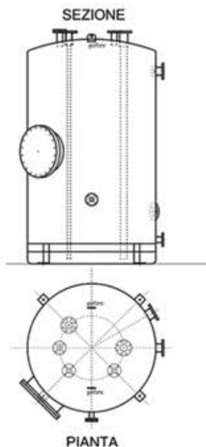
SERBATOIO VERTICALE ESEMPIO DI POSSIBILE ESECUZIONE
